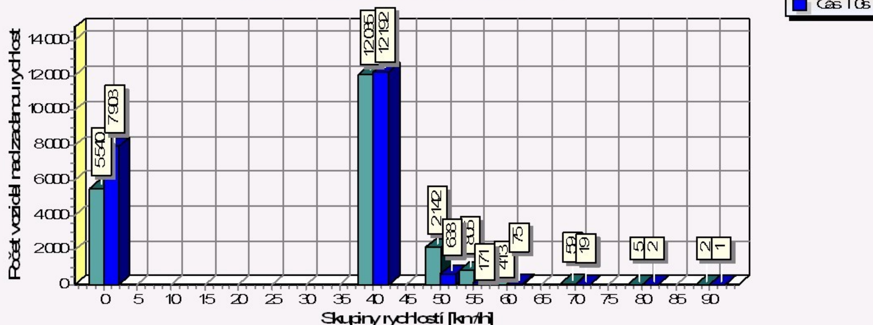
Graf rychlosti vozidel před zařízením v časech T0 a T5s za období od 01.04.23 00:00 do 30.04.23 23:59
