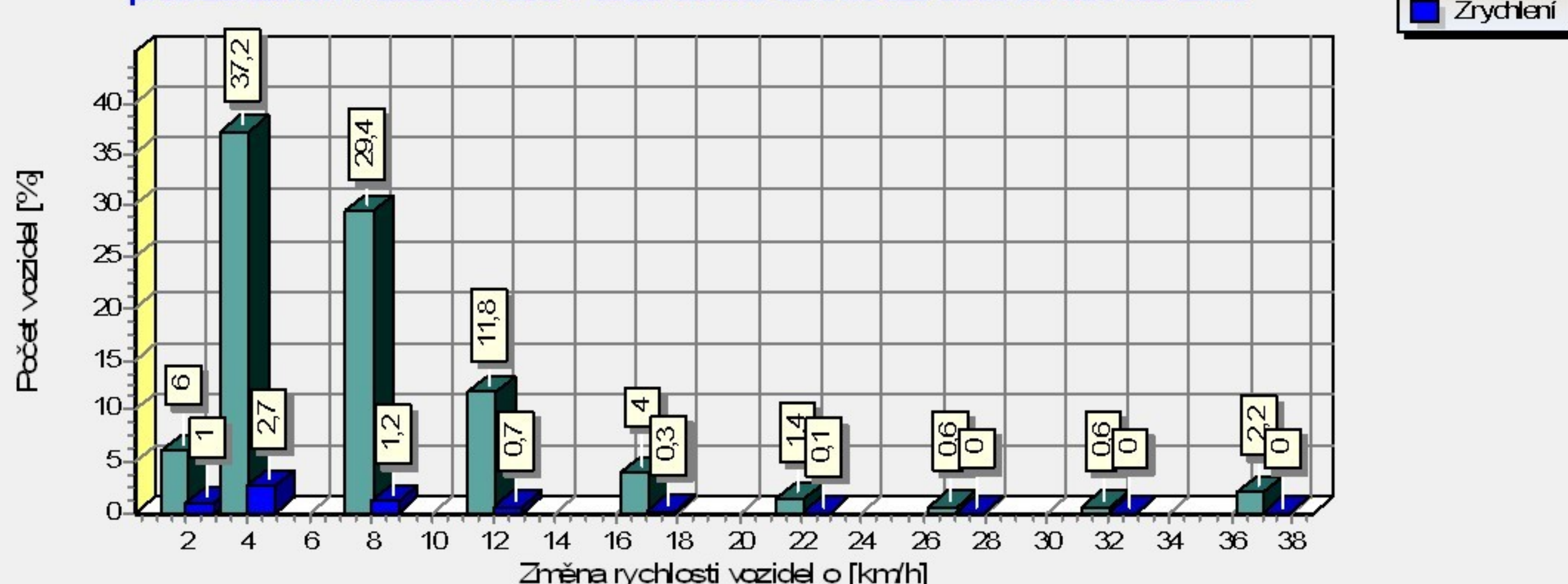
Graf velikosti změny rychlosti vozidel před zařízením v časech T 0s a T-5s za období od 01.04.23 00:00 do 30.04.23 23:59
