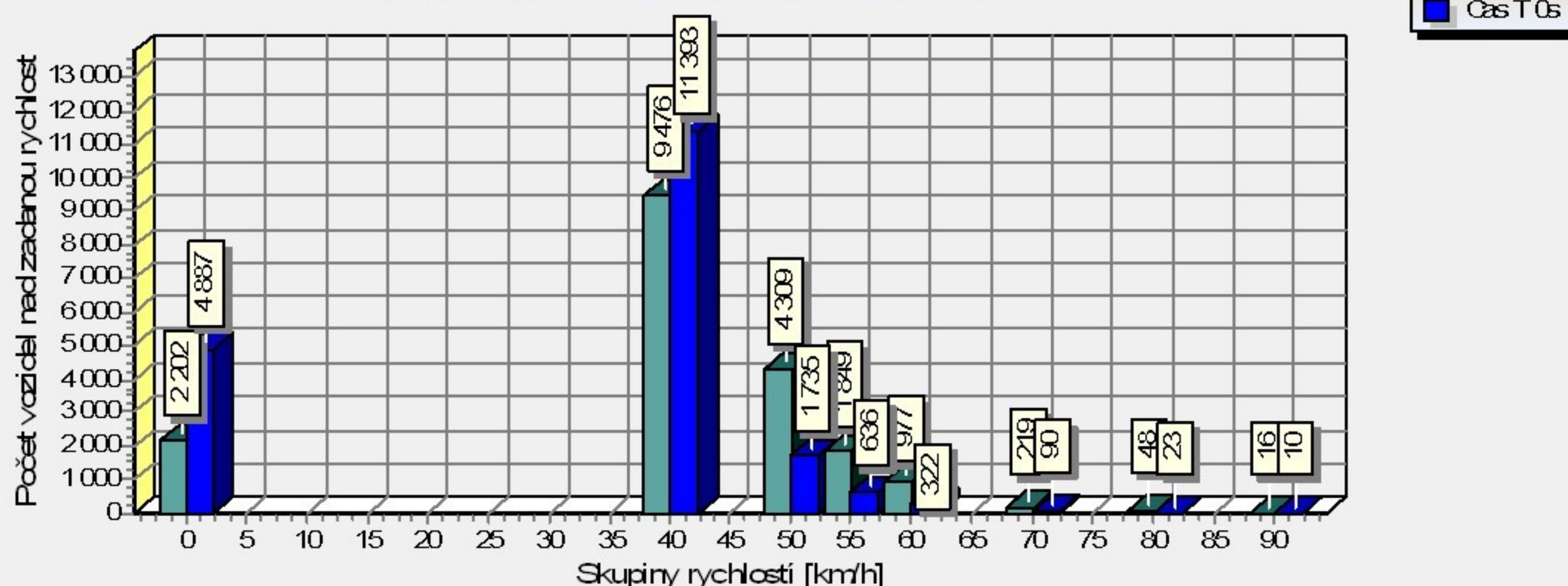
Graf rychlosti vozidel před zařízením v časech T 0s a T-5s za období od 01.04.23 00:00 do 30.04.23 23:59
